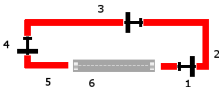
图 9.15: 起落航线
